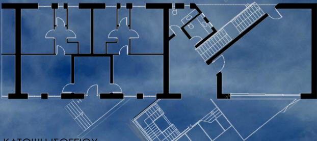
ΚΑΤΟΨΗ ΙΣΟΓΕΙΟΥ
